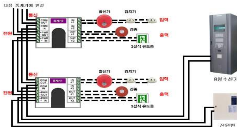
[ 그림 1-56 ] 분산형 중계기 계통배선
