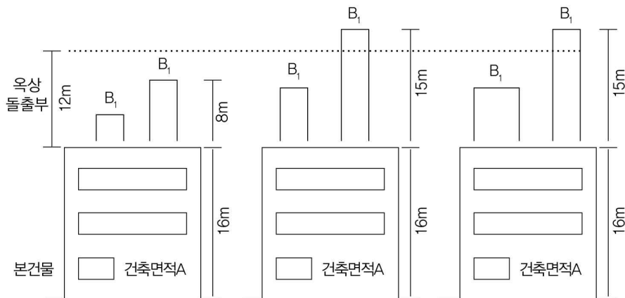
[ 그림 3-15 ] 옥상부분의 면적에 따른 건축물의 높이 산정
