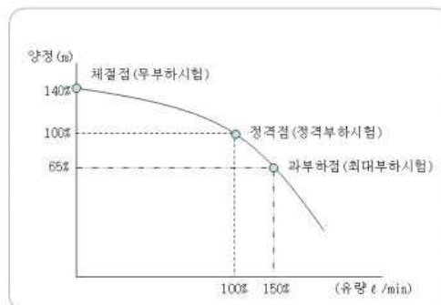
[ 그림 2-29 ] 소방펌프의 특성곡선
