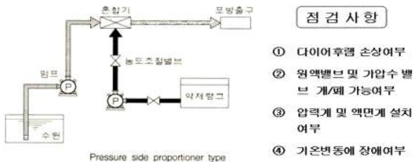
[ 그림 2-86 ] 프레저사이드프로포셔너 방식
