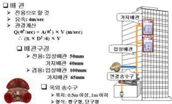
[ 그림 2-31 ] 배관 및 송수구
