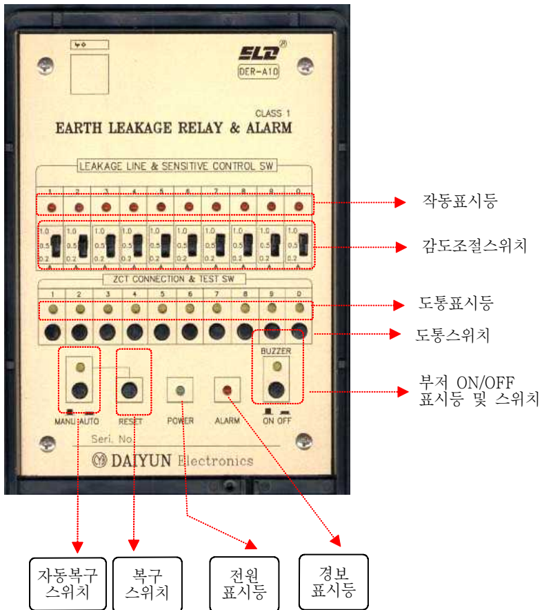
[ 그림 1-72 ] 누전경보기의 표시등 및 스위치
