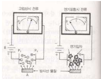
[ 그림 1-22 ] 이온화식감지기의 회로구성
