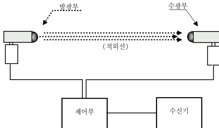
[ 그림 1-26 ] 광전식분리형감지기
