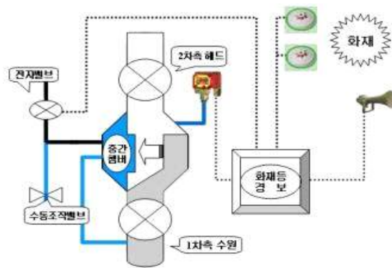
[ 그림 2-53 ] 준비작동식밸브 교차회로방식
