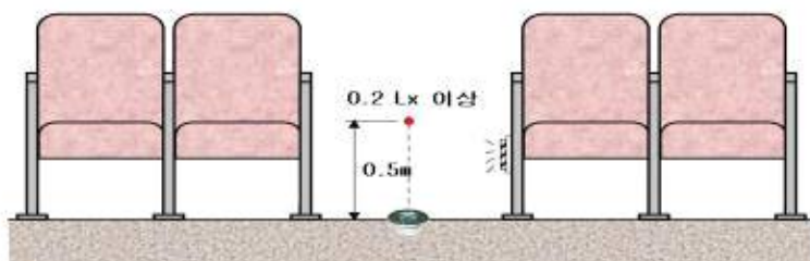
[ 그림 1-90 ] 객석유도등의 설치기준
