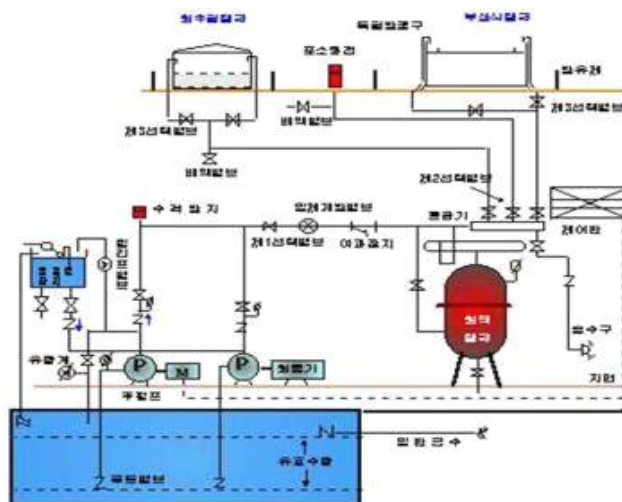
[ 그림 2-87 ] 고정포 방출설비
