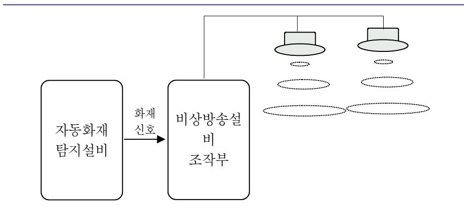
[ 그림 1-80 ] 비상방송설비의 작동흐름도
