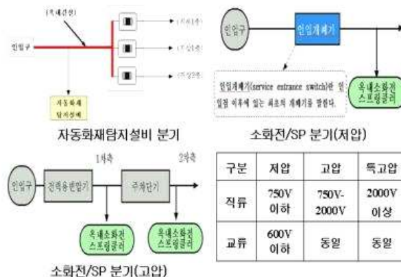
[ 그림 2-38 ] 상용전원 분기방식
