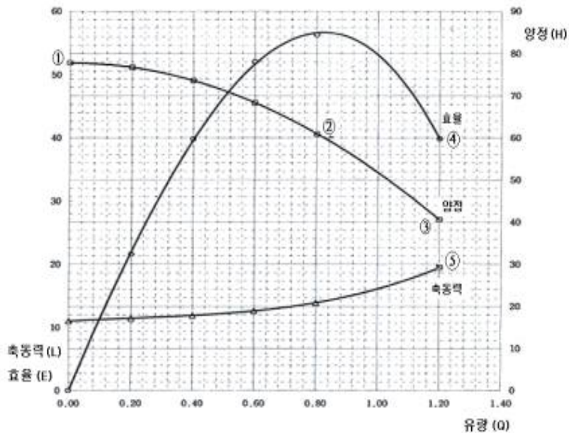
[ 그림 2-34 ] 양정계산과 압력세팅
