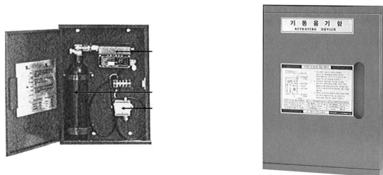
[ 그림 2-110 ] 기동용기함
