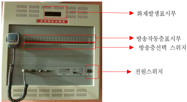
[ 그림 1-81 ] 비상방송설비의 스위치 및 표시등
