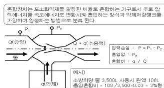
[ 그림 2-80 ] 포소화약제 혼합장치
