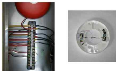
[ 그림 1-52 ] 종단저항 설치(발신기세트함 및 종단감지기)
