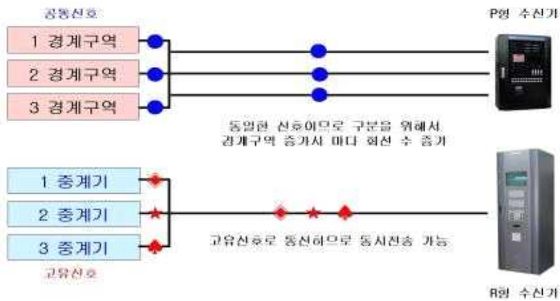
[ 그림 1-5 ] 공통신호와 고유신호의 구분
