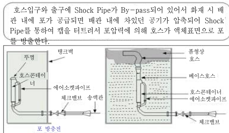
[ 그림 2-93 ] 반표면하 방식
