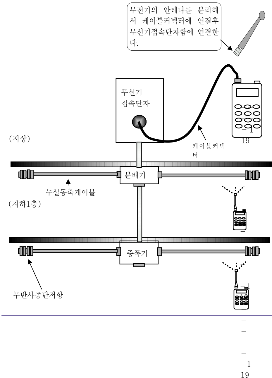
[ 그림 1-105 ] 무선통신보조설비의 구성
