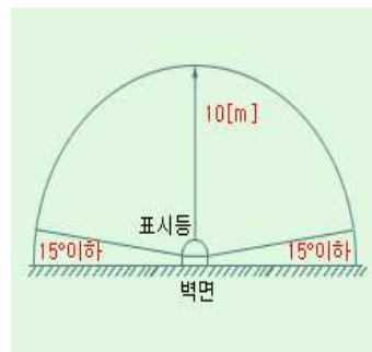
[ 그림 1-42 ] 표시등의 식별범위
