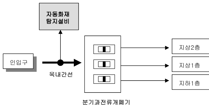
[ 그림 1-112 ] 자동화재탐지설비 상용전원의 분기
