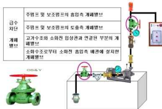
[ 그림 2-19 ] 급수차단 밸브 구분
