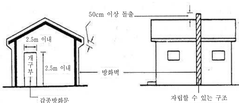
[ 그림 3-21 ] 방화벽 설치
