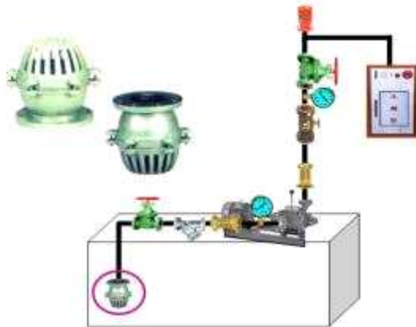
[ 그림 2-18 ] 가압송수장치 펌프방식
