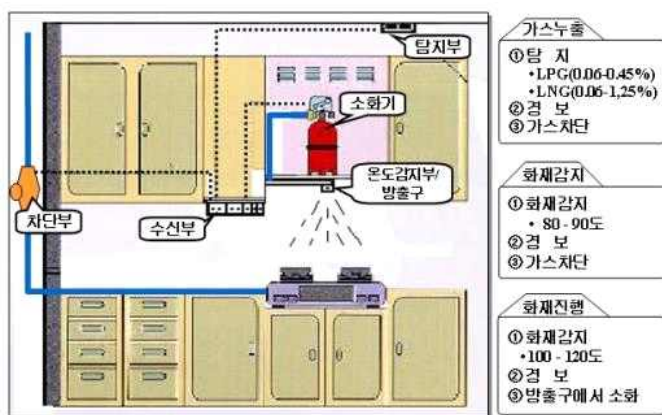
[ 그림 2-7 ] 주거용 주방자동소화장치
