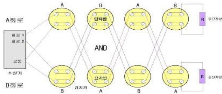
[ 그림 1-2 ] 자동소화설비 화재감지기용 회로는 교차회로
