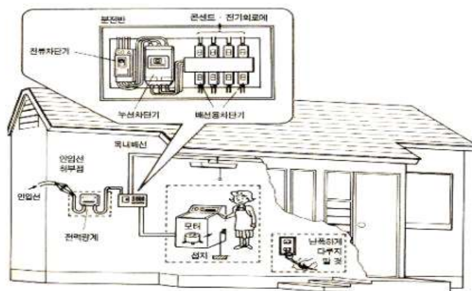
[ 그림 2-36 ] 상용전원 결선도
