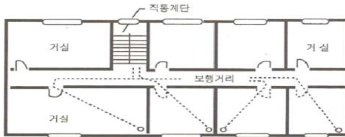
[ 그림 3-28 ] 직통계단까지 보행거리
