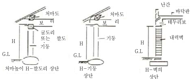
[ 그림 3-18 ] 처마높이 산정
