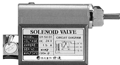
[ 그림 2-111 ] 기동용 솔레노이드 밸브
