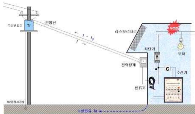
[ 그림 1-70 ] 누전경보기 설치구성도
