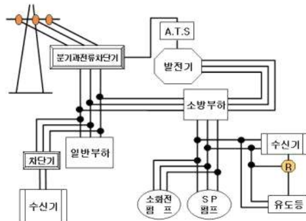
[ 그림 2-37 ] 소방시설 전원 결선도
