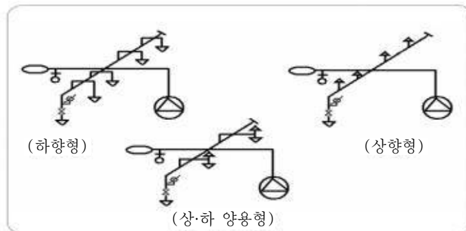
[ 그림 2-63 ] 헤드설치방법
