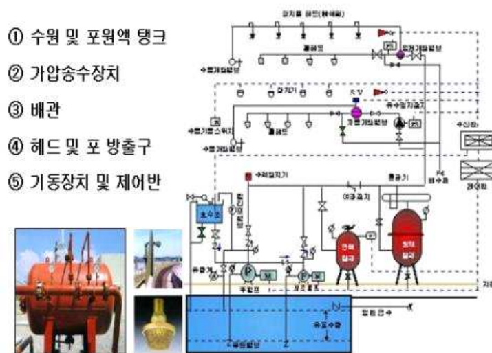
[ 그림 2-76 ] 고포소화설비 구성요소
