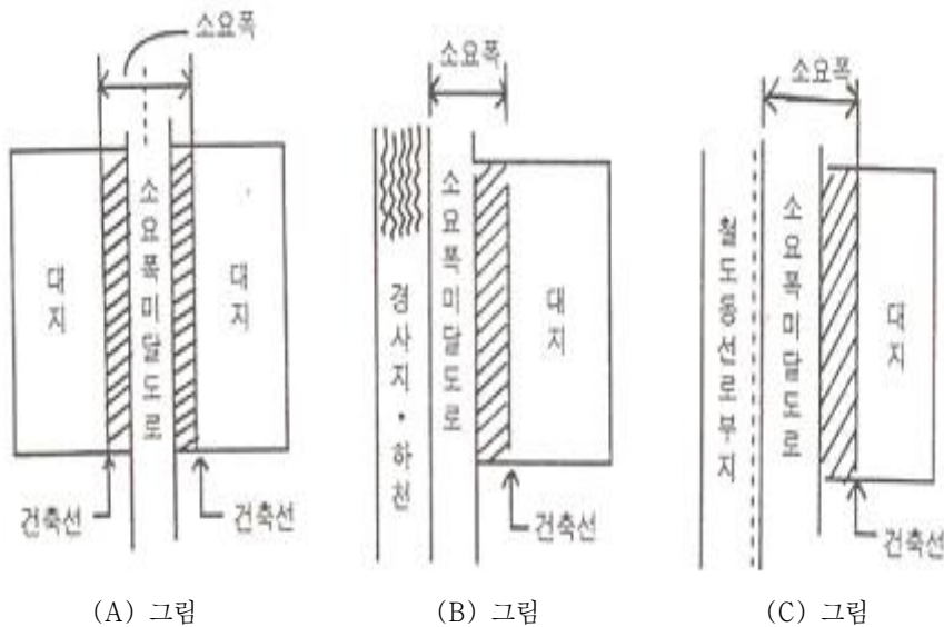
[ 그림 3-5 ] 대지면적의 산정방법(2)
