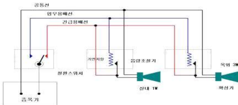
[ 그림 1-82 ] 3선식 배선의 결선
