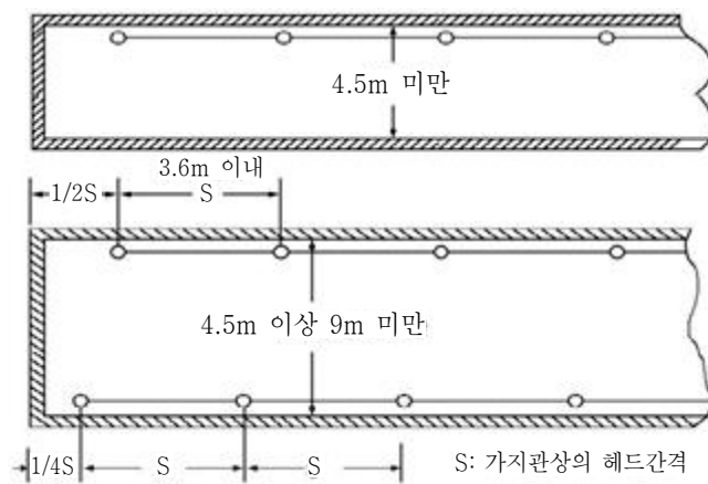
[ 그림 2-69 ] 측벽형 헤드설치
