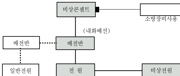
[ 그림 1-100 ] 비상콘센트설비의 구성
