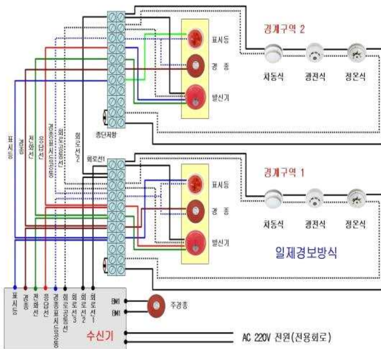
[ 그림 1-54 ] 여러 경계구역의 연결
