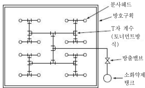
[ 그림 2-120 ] 토너먼트 배관의 설치 예
