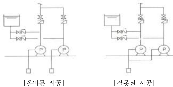
[ 그림 2-23 ] 물울림장치와 흡수배관의 설치 예
