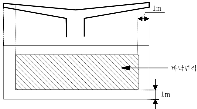
[ 그림 3-8 ] 벽·기둥의 구획이 없는 건축물의 바닥면적 산정방법
