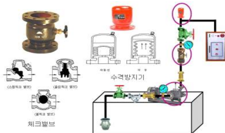
[ 그림 2-21 ] 체크밸브와 수격방지기
