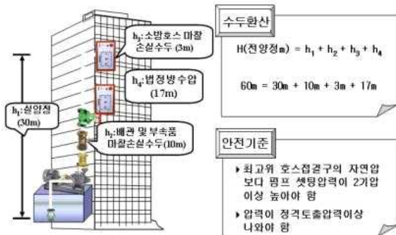
[ 그림 2-33 ] 양정계산과 압력세팅
