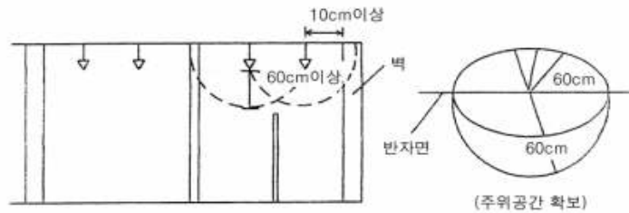
[ 그림 2-65 ] 헤드설치 살수반경
