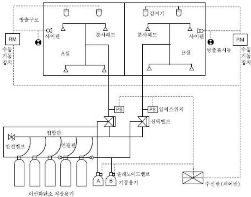
[ 그림 2-104 ] 이산화탄소 소화설비 계통도
