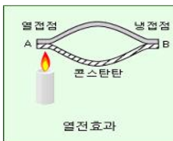
[ 그림 1-12 ] 제백효과
