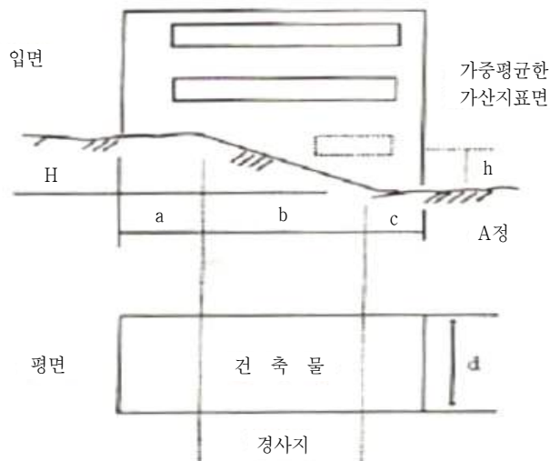
[ 그림 3-13 ] 지표면의 산정
