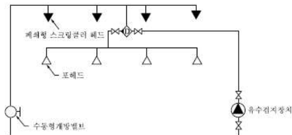
[ 그림 2-77 ] 폐쇄형 스프링클러헤드 감지
