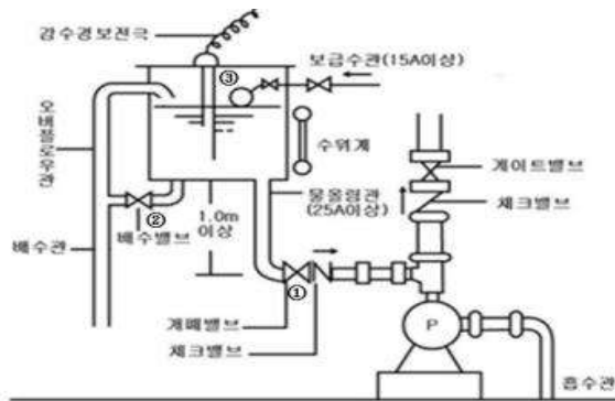
[ 그림 2-47 ] 자가발전설비 물올림 장치 점검
