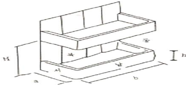
[ 그림 3-9 ] 노대등의 바닥면적 산정방법(1)
