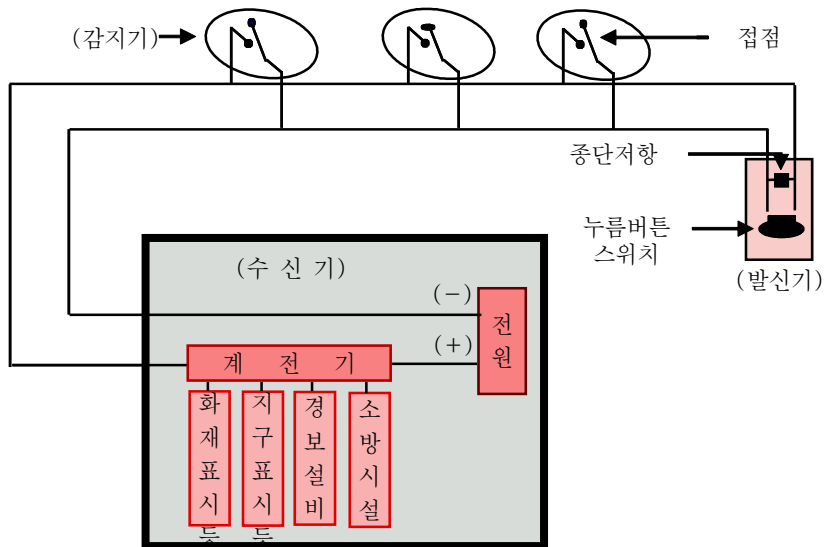
[ 그림 1-4 ] 자동화재탐지설비의 회로 간략도
