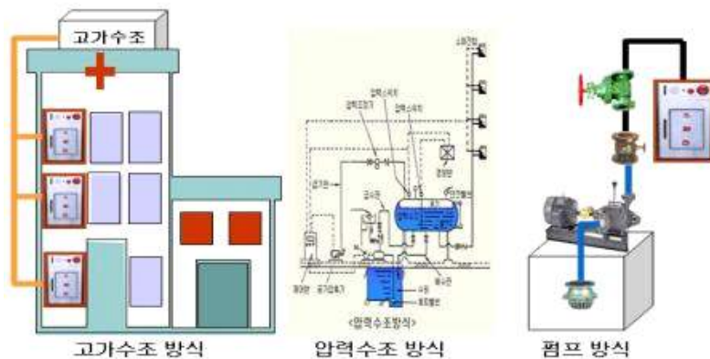
[ 그림 2-17 ] 가압송수장치 종류
