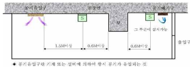
[ 그림 1-35 ] 연기감지기의 설치위치
