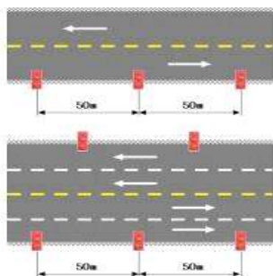
[ 그림 1-43 ] 터널 설치기준과 보행거리 초과시 추가설치
