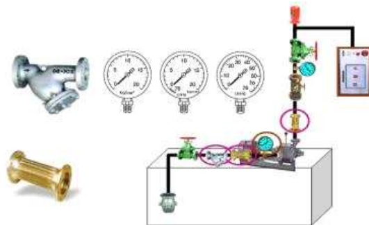
[ 그림 2-20 ] 흡입측 배관 부속품 및 밸브류
