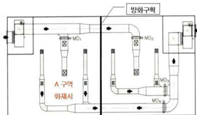
[ 그림 2-128 ] 동일실 급배기 방식
