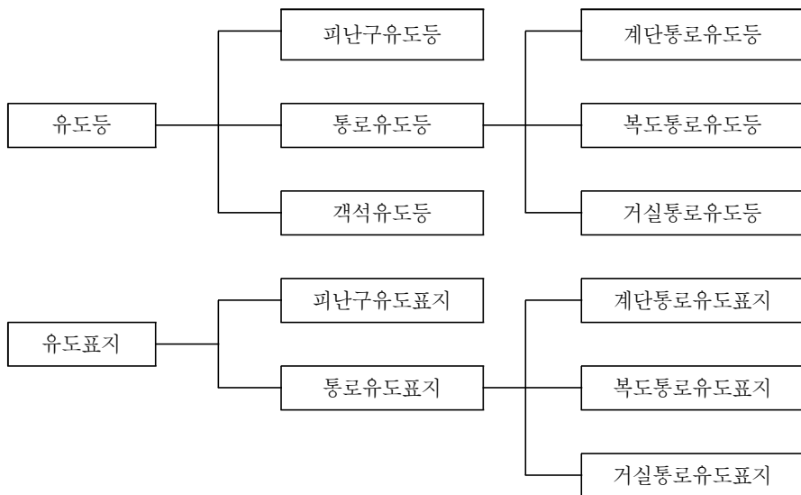
[ 그림 1-85 ] 유도등의 분류
