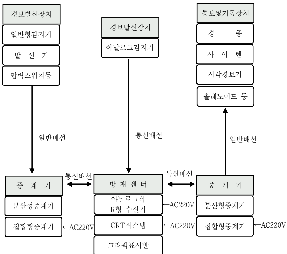
[ 그림 1-58 ] 아날로그식 감지기를 사용하는 경우
