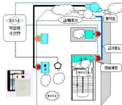
[ 그림 2-134 ] 부속실 제연설비 작동
