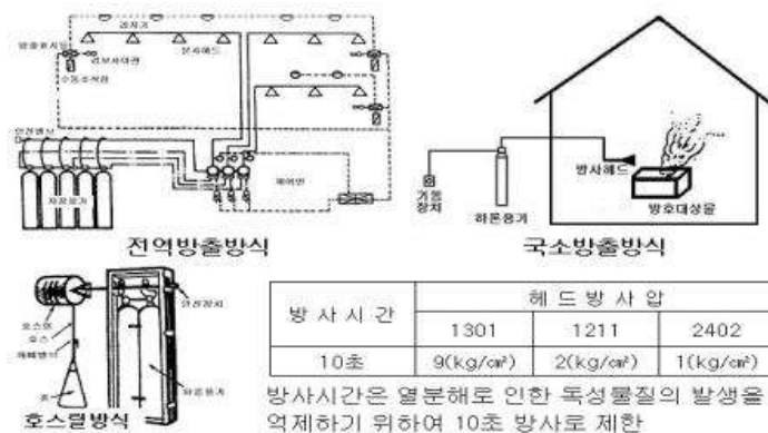
[ 그림 2-117 ] 소화약제 방출방식
