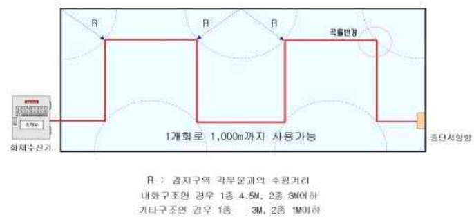
[ 그림 1-37 ] 정온식감지선형감지기 설치기준
