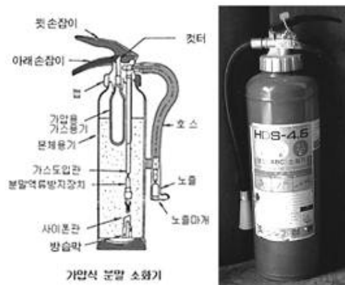
[ 그림 2-4 ] 가압식 분말소화기 구조
