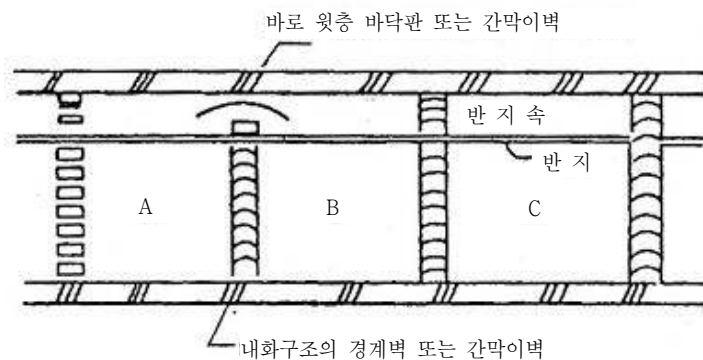
[ 그림 3-22 ] 경계벽 및 간막이벽의 설치방법
