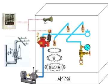
[ 그림 2-49 ] 스프링클러설비 구조 및 작동
