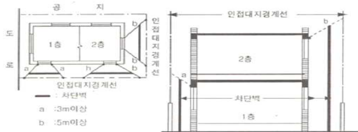
[ 그림 3-23 ] 차단벽 설치
