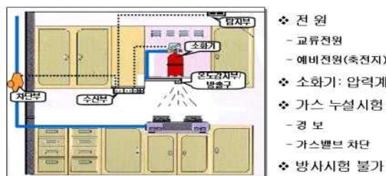
[ 그림 2-13 ] 주거용 주방자동소화장치 점검
