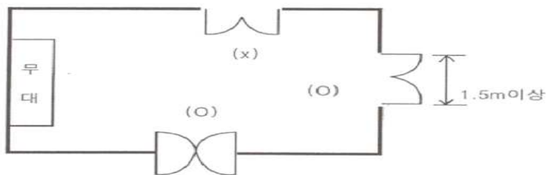
[ 그림 3-29 ] 출구의 문 설치기준
