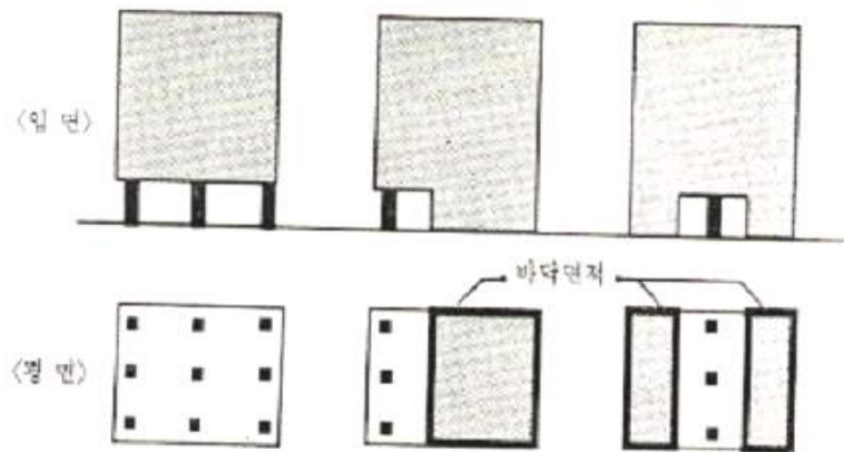
[ 그림 3-11 ] 피로티의 바닥면적 산정방법
