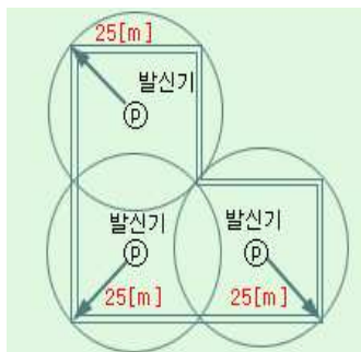
[ 그림 1-41 ] 발신기의 설치거리
