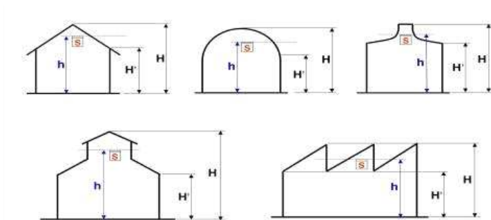
[ 그림 1-33 ] 건축물별 감지기의 설치높이 산정방법
