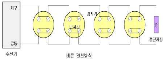
[ 그림 1-53 ] 감지기 배선 송배선방식
