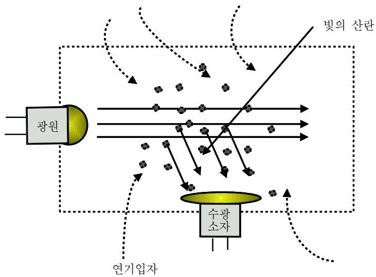
[ 그림 1-24 ] 산란광식의 감지원리
