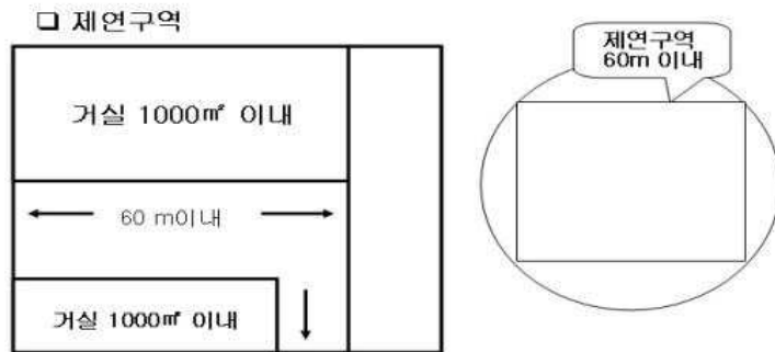
[ 그림 2-132 ] 제연구역 설정
