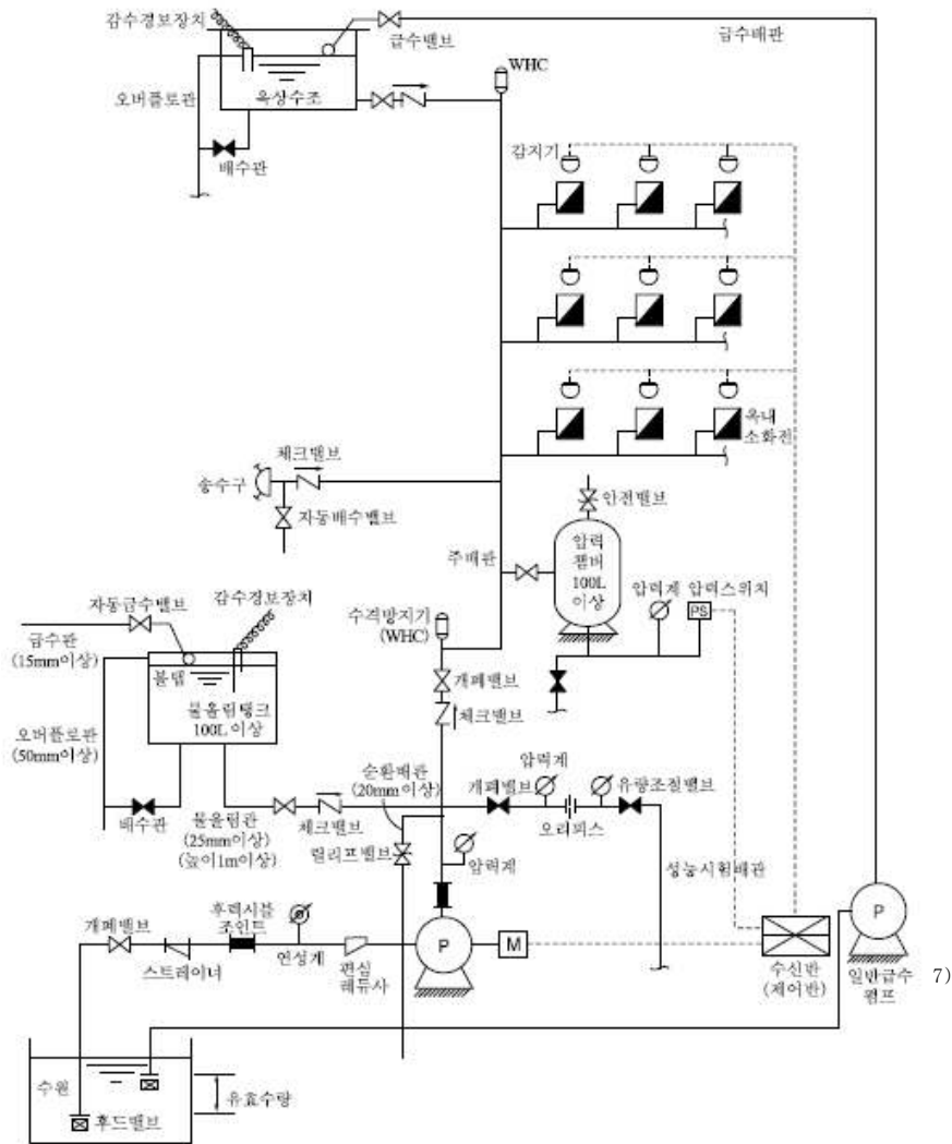
[ 그림 2-14 ] 옥내소화전 계통도
