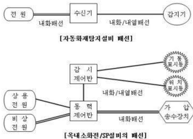
[ 그림 2-40 ] 소방시설별 내화/내열배선 방식
