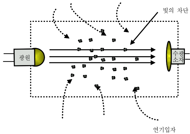
[ 그림 1-23 ] 감광식의 감지형태
