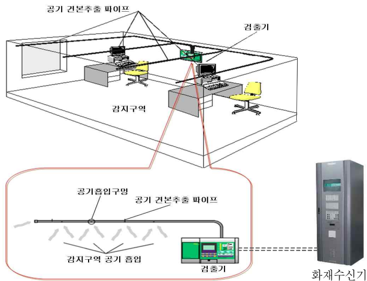
[ 그림 1-27 ] 광전식 공기흡입형감지기의 구성
