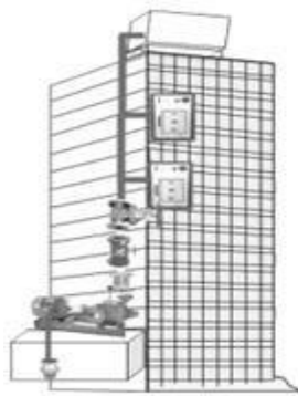
[ 그림 2-15 ] 옥내소화전 수원산정
