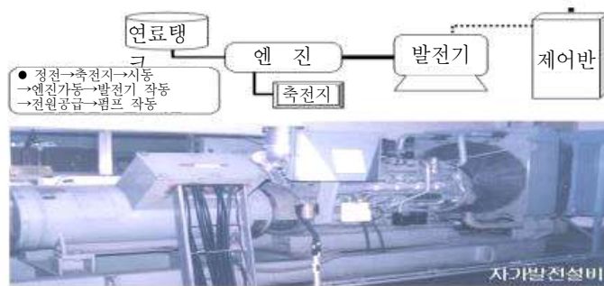
[ 그림 2-41 ] 자가발전설비
