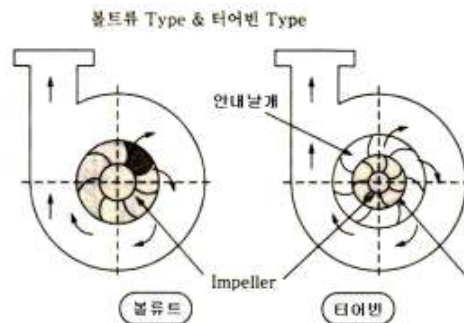
[ 그림 2-25 ] 소방용 원심펌프
