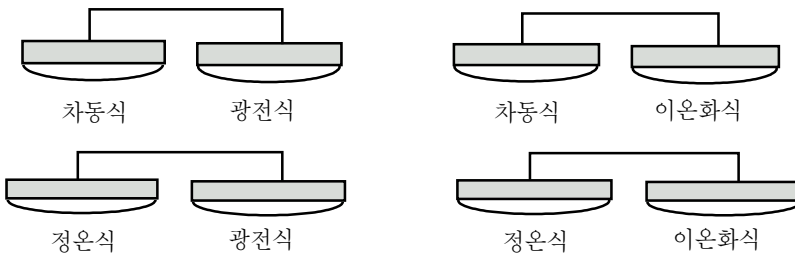
[ 그림 1-30 ] 열연복합형감지기의 구성
