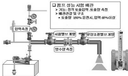
[ 그림 2-28 ] 펌프성능시험 배관
