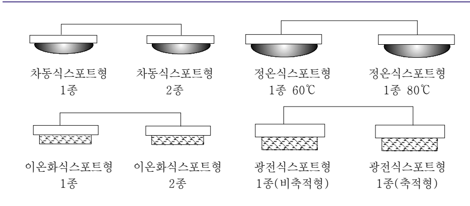
[ 그림 1-31 ] 다신호식감지기의 구성
