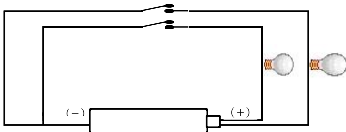
[ 그림 1-51 ] 공통선 배선
