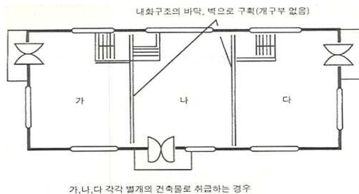
[ 그림 3-25 ] 별개의 건축물
