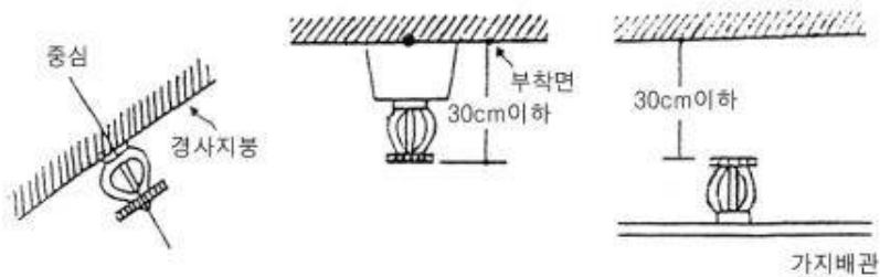
[ 그림 2-66 ] 헤드설치 살수방법
