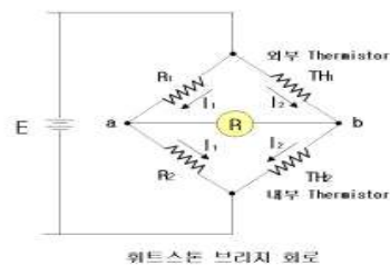
위트스톤 브리지 회로
