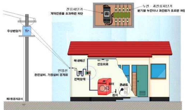
[ 그림 1-109 ] 일반주택의 옥내·외 배선
