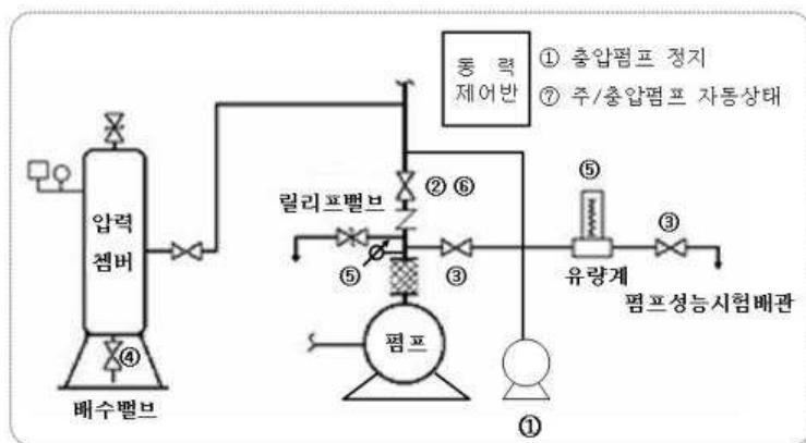
[ 그림 2-45 ] 펌프성능시험 방법
