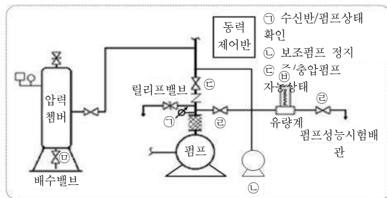
[ 그림 2-30 ] 펌프성능시험 방법
