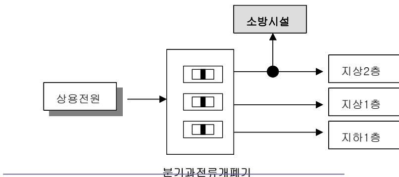
[ 그림 1-110 ] 소방시설 상용전원의 분기(×)
