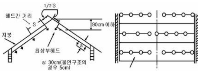
[ 그림 2-67 ] 경사지붕의 헤드설치
