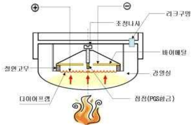
[ 그림 1-20 ] 보상식감지기 구조
