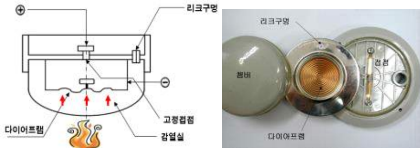
[ 그림 1-6 ] 차동식스포츠형 감지기 구조
