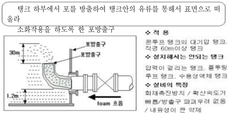
[ 그림 2-92 ] 표면하 주입구
