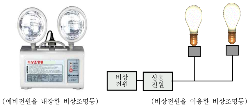
[ 그림 1-98 ] 비상조명등의 형태
