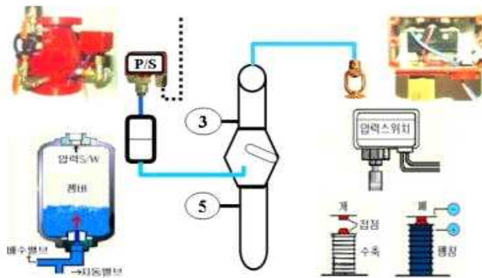
[ 그림 2-51 ] 압력스위치와 리타딩 챔버
