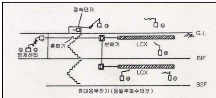
[ 그림 1-107 ] 무선통신보조설비의 사용
