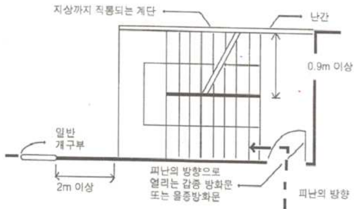
[ 그림 3-37 ] 옥외피난계단의 구조
