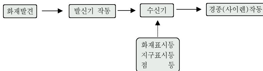
[ 그림 1-77 ] 비상벨설비의 작동흐름도
