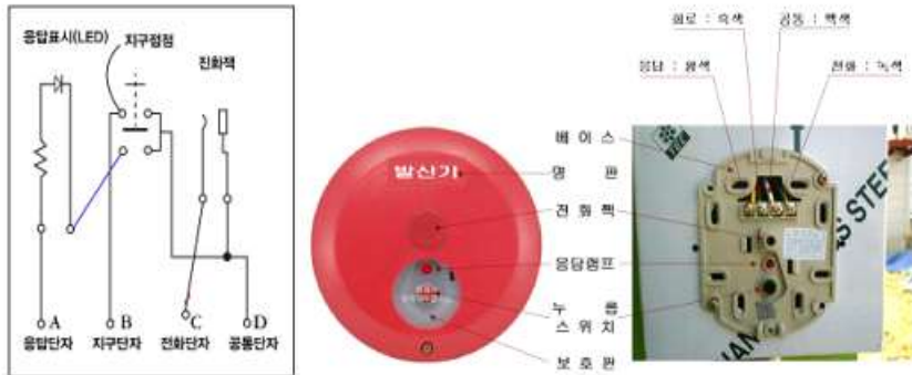
[ 그림 1-40 ] 발신기 구성
