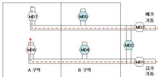
[ 그림 2-131 ] 화재시 제연설비로 전환
