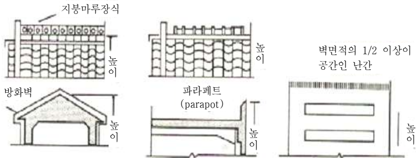
[ 그림 3-16 ] 옥상돌출물이 있는 건축물의 높이 산정
