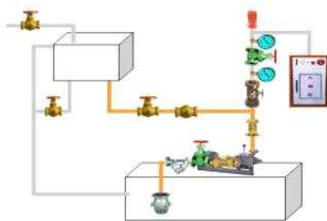
[ 그림 2-22 ] 물울림 장치 구조
