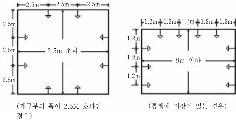
[ 그림 2-69 ] 측벽형 헤드설치
