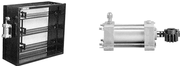
[ 그림 2-114 ] 댐퍼와 피스톤릴리저
