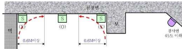
[ 그림 1-34 ] 벽 및 보로부터의 감지기의 설치위치
