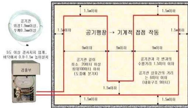
[ 그림 1-36 ] 공기관식 감지기의 설치기준
