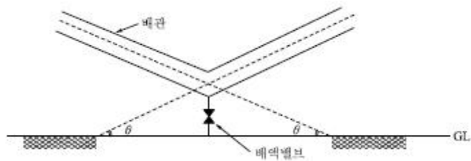
[ 그림 2-96 ] 송액관의 경사와 배액밸브
