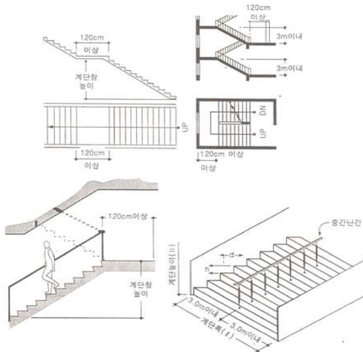
[ 그림 3-33 ] 계단의 설치기준
