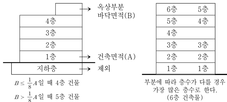
[ 그림 3-19 ] 건축물의 층수산정
