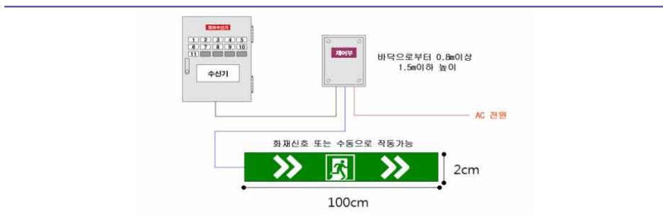
[ 그림 1-92 ] 광원점등방식 피난유도선 구성도
