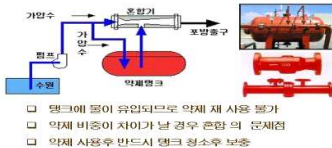
[ 그림 2-84 ] 격막이 없는 방식
