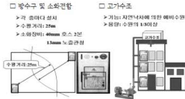
[ 그림 2-32 ] 소화전함 설치
