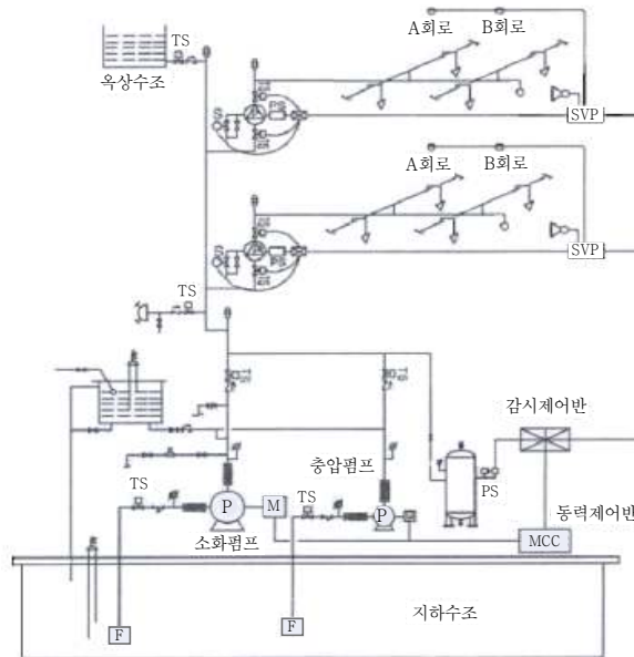
[ 그림 2-48 ] 준비작동식 스프링클러설비 계통도
