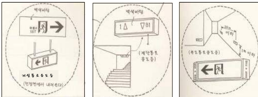
[ 그림 1-89 ] 통로유도등의 설치 기준
