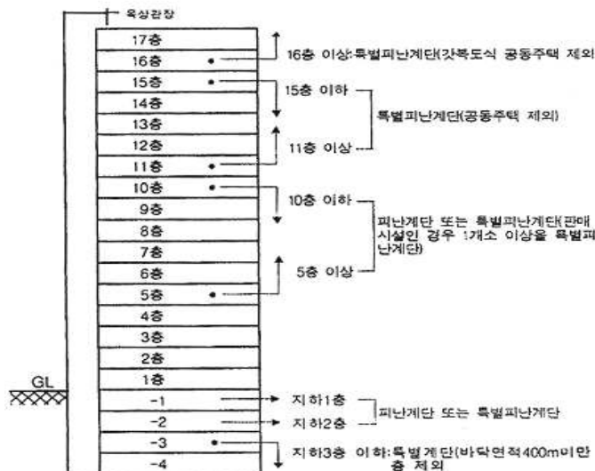
[ 그림 3-35 ] 피난계단 설치기준
