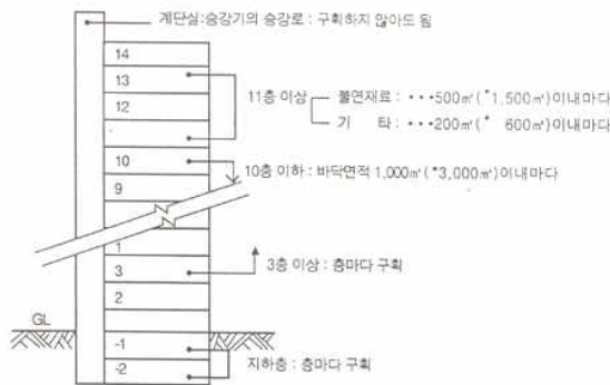
[ 그림 3-20 ] 방화구획 설치기준
