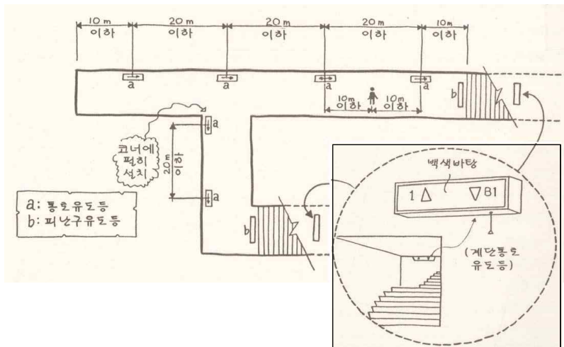
[ 그림 1-88 ] 통로유도등 및 피난구유도등의 설치기준
