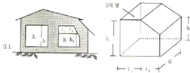
[ 그림 3-17 ] 반자 높이 산정
