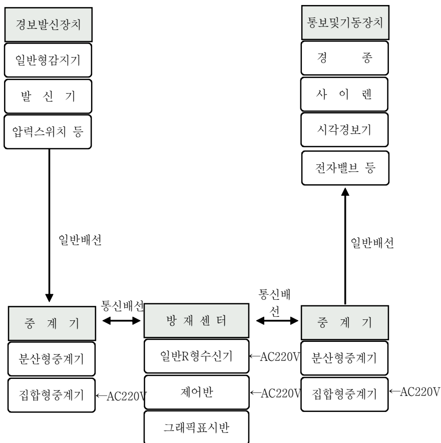
[ 그림 1-57 ] 중계기를 사용한 R형 설비
