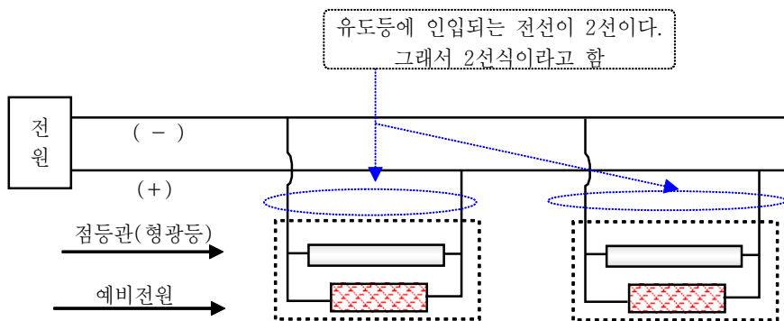
[ 그림 1-94 ] 2선식 유도등의 배선
