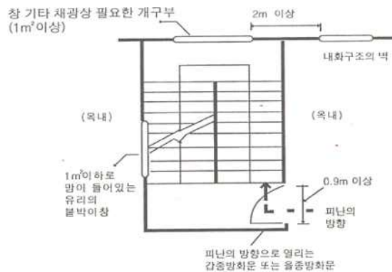
[ 그림 3-36 ] 옥내피난계단의 구조
