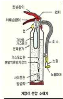
[ 그림 2-9 ] 가압식 분말소화기 점검
