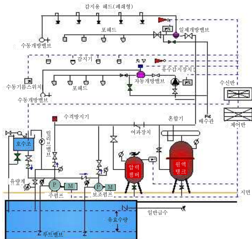
[ 그림 2-88 ] 포헤드설비 방식
