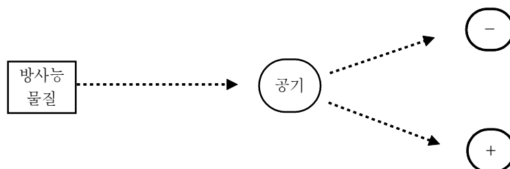
[ 그림 1-21 ] 방사능 물질에 의한 공기의 이온화
