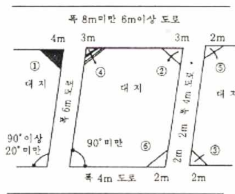
[ 그림 3-6 ] 가각정리의 예시
