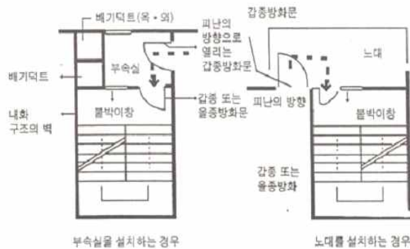
[ 그림 3-38 ] 특별피난계단의 구조
