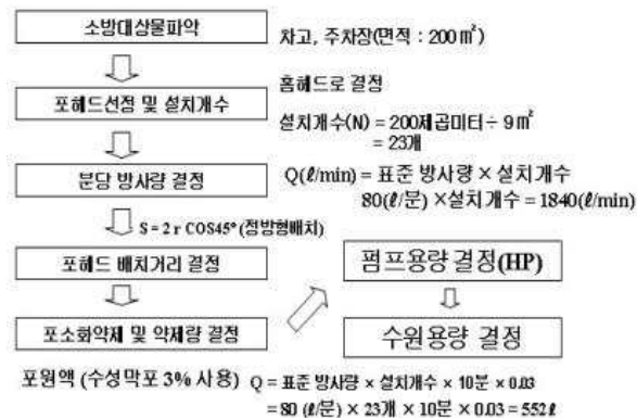
[ 그림 2-100 ] 포헤드 설계방식 검토
