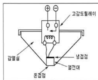
[ 그림 1-13 ] 열전대식감지기
