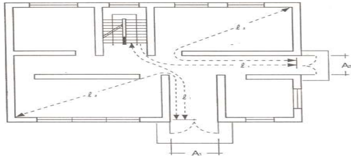
[ 그림 3-30 ] 거실 및 직통계단에서 옥외로의 출구까지 보행거리 기준
