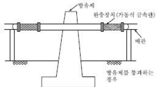
[ 그림 2-97 ] 방유제의 배관 연결
