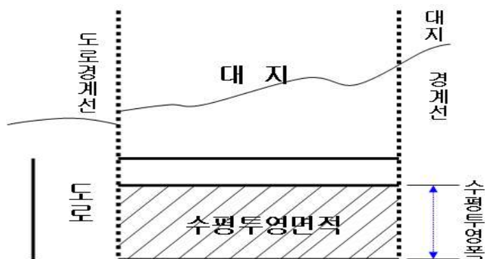
[ 그림 3-4 ] 대지면적의 산정방법(1)
