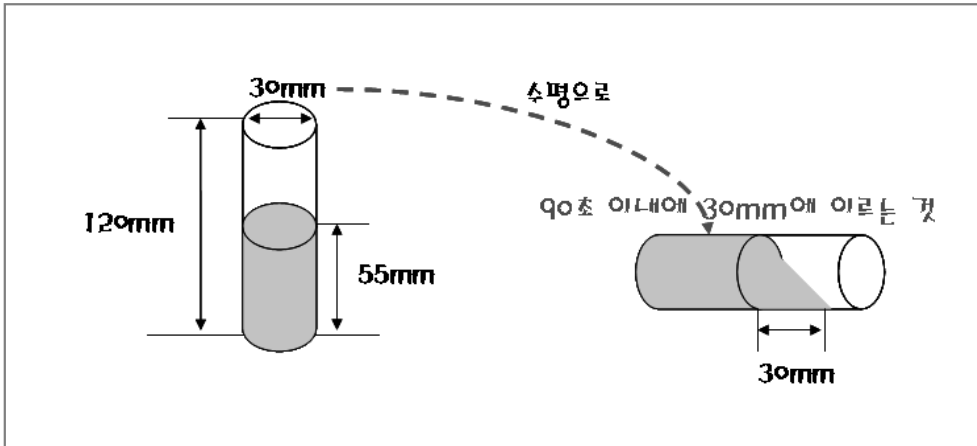
[그림 4-1] 액상 시험방법
