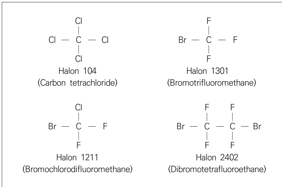
[그림 2-2] 대표적인 할로겐화합물 소화약제의 구조식
