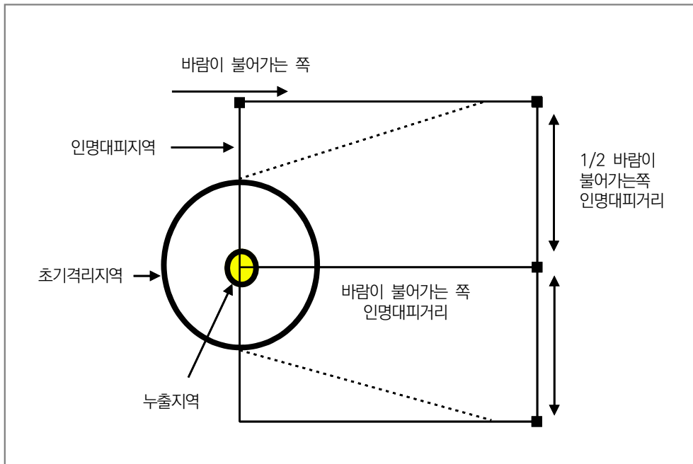
[그림 4-6] 인명대피거리
